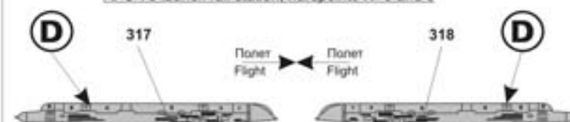
Пусковое устройство АПУ-73, точки подвеса 5 и 6 APU-73 launch rail station, hardpoints № 5 and 6
