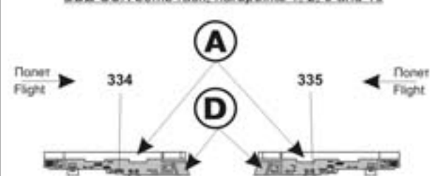
Балочный держатель БДЗ-УСК, точки подвеса 1, 2, 9 и 10 BDZ-USK bomb rack, hardpoints 1, 2, 9 and 10
