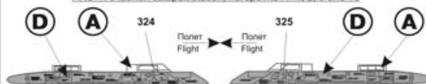
Пусковое устройство АКУ-470, точки подвеса 1, 2, 9 и 10 AKU-470 launch catapult station, hardpoints № 1, 2, 9 and 10
