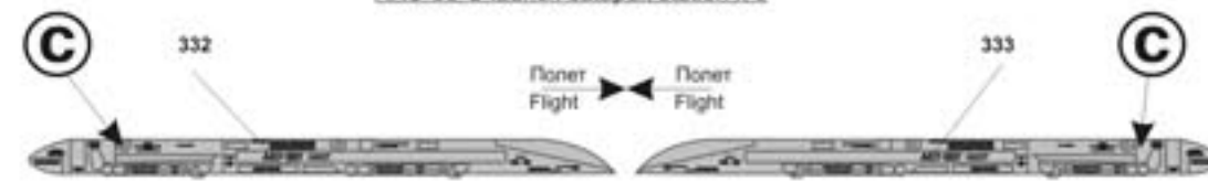
Пусковое устройство АКУ-58-У x 6 AKU-58-U launch catapult station x 6
