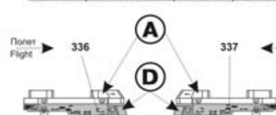
Балочный держатель БДЗ-УСК с переходной балкой, точки подвеса 3 и 4 BDZ-USK bomb rack with adapter for hardpoints 3 and 4
